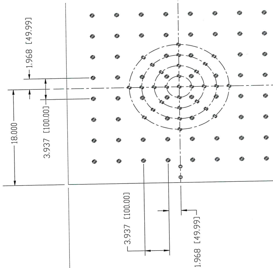
Rys. 2 Rozstaw otworów stołu ślizgowego, z którym system musi być kompatybilny.
